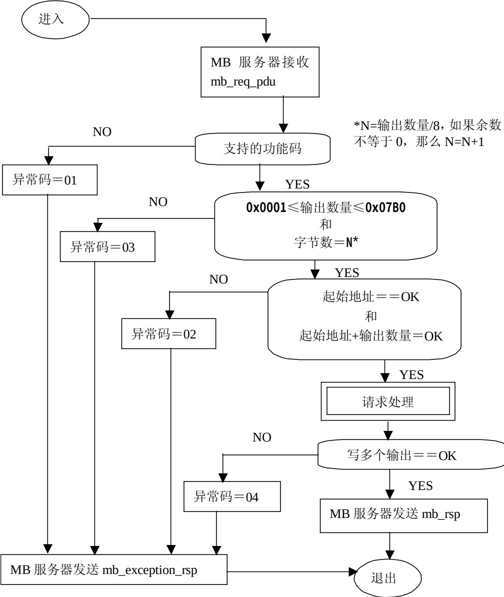
图 16: 写多个输出的状态图
