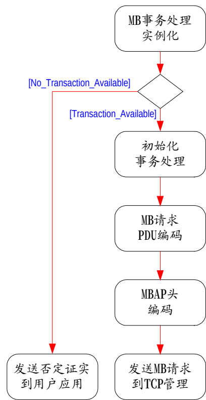
图 12：请求生成操作示意图
