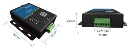
产品尺寸
